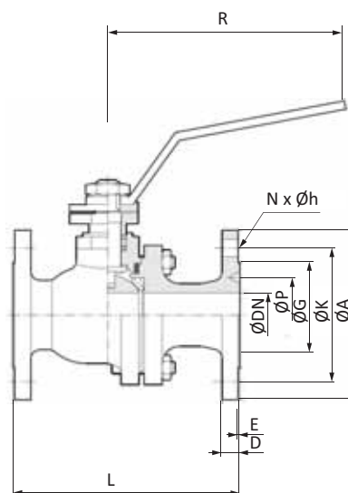
Размер 1/2"-1 1/2"
